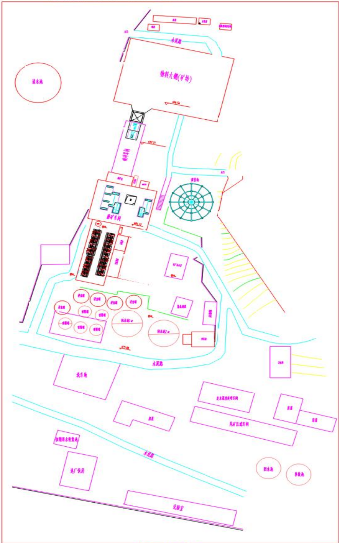
附图二 选厂平面布置图
