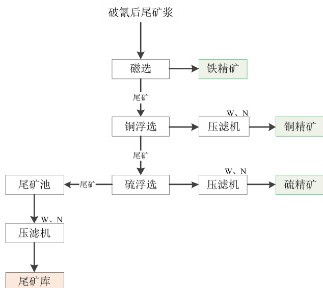
图 4-2 本项目多金属回收生产工艺及产污环节示意图
