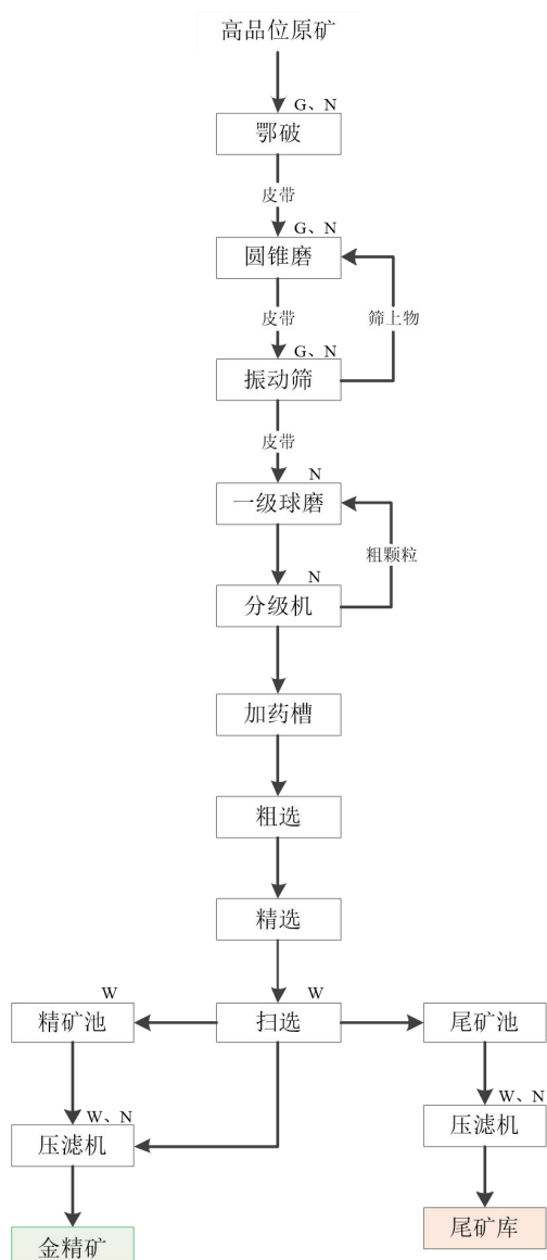
图 4-1 项目金浮选生产工艺及产污环节示意图
