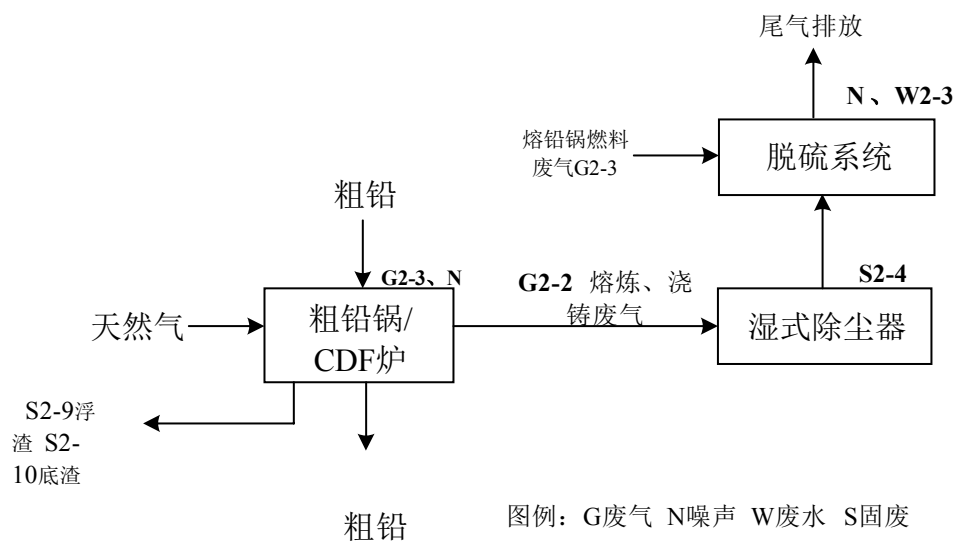
图 4-4 初步火法精炼工艺流程及产污环节图
