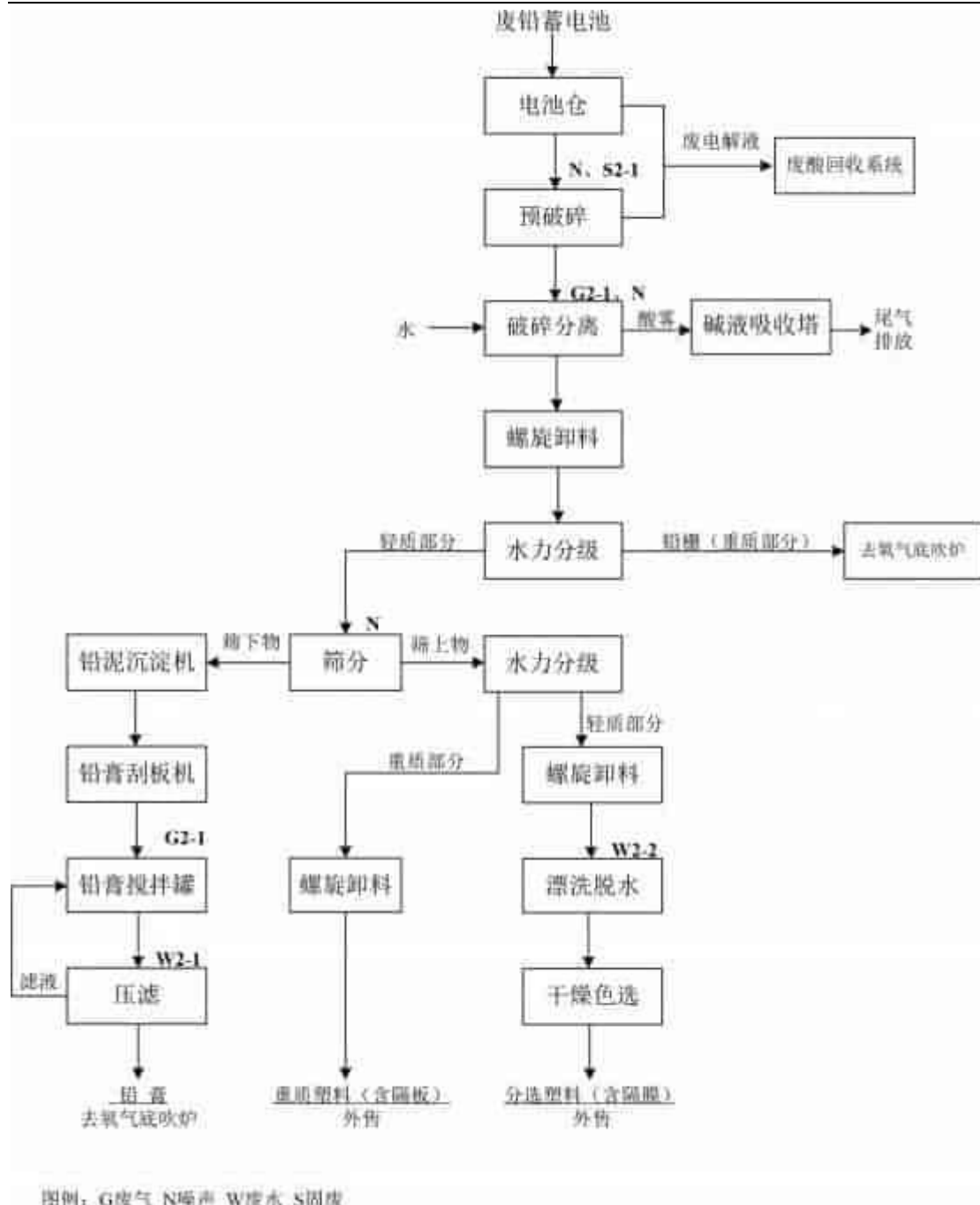
图4-1 废铅蓄电池拆解生产工艺及产污环节示意图
