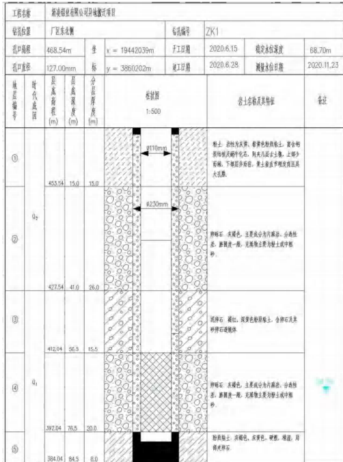
图3-2 厂区钻孔 ZK1 柱状图
