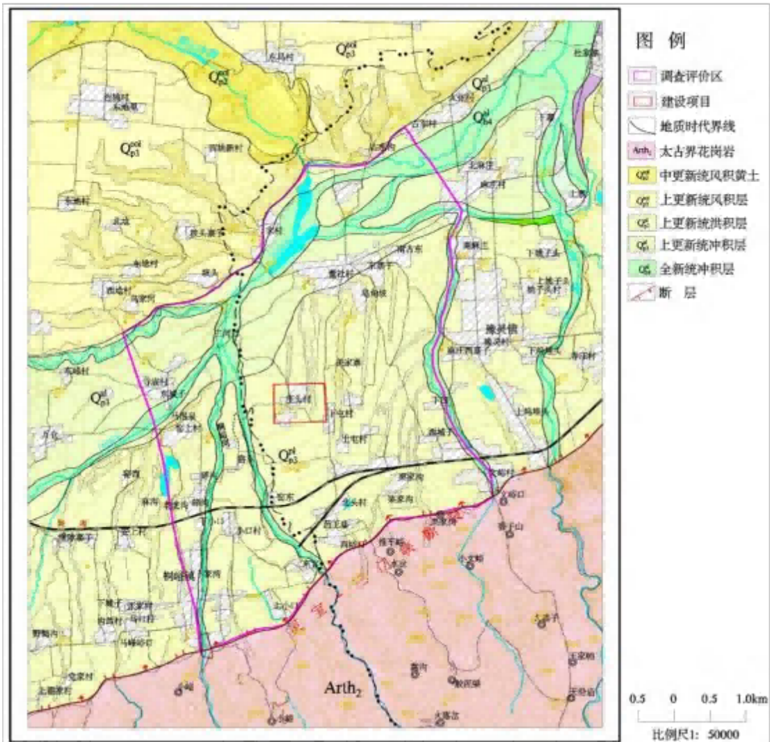
图3-1 区域地质图
