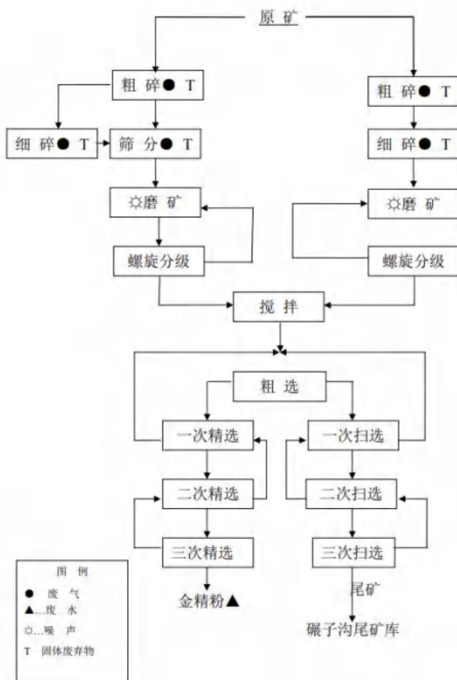
图 4-6 崑鑫选厂工艺流程
