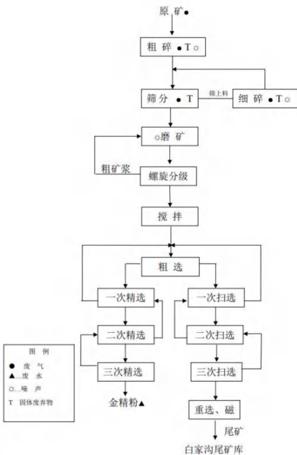
图 4-5 枪马一选厂工艺流程
