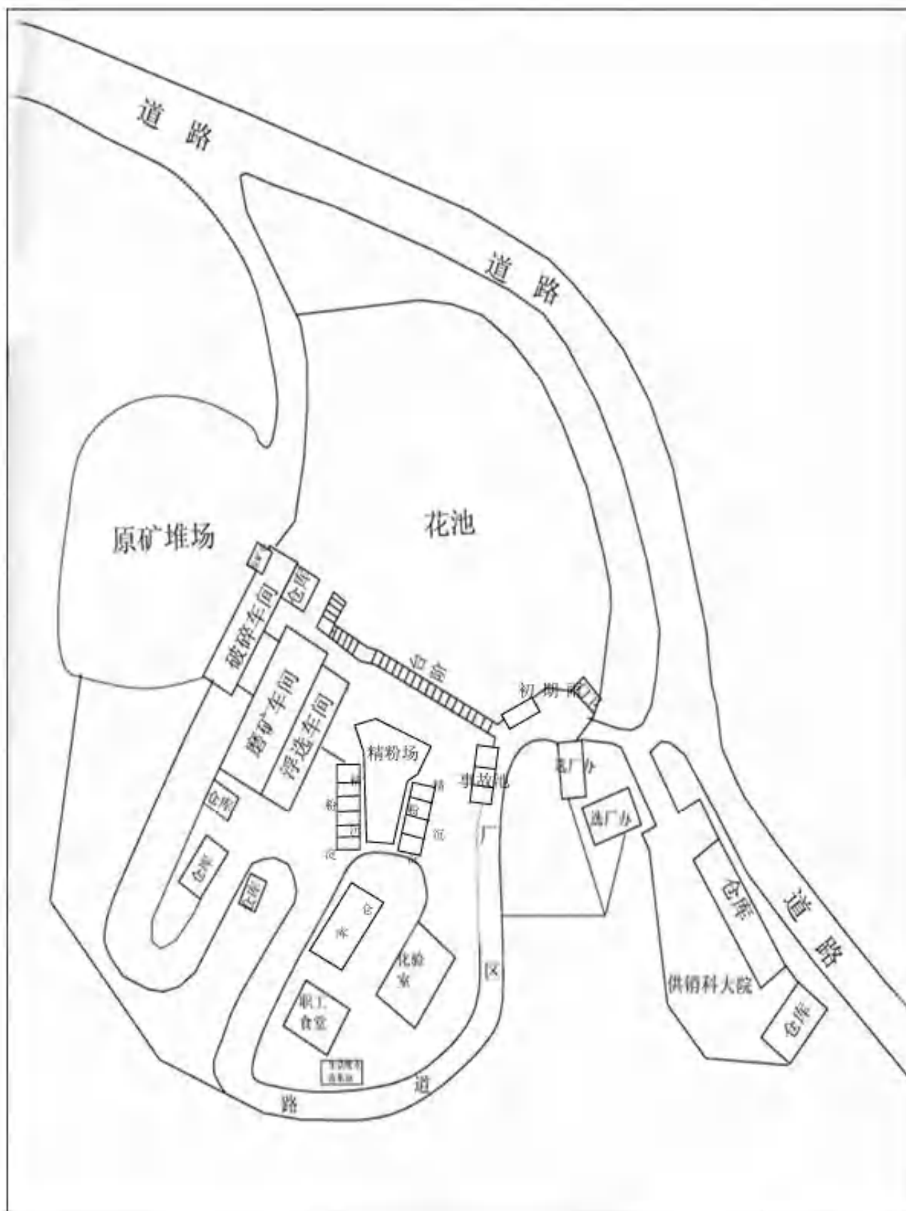
附图一 枪马一选厂平面布置图
