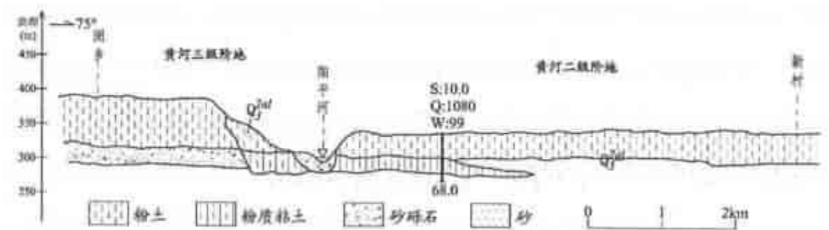
图 3.1-1 阌乡——新村地质剖面图
