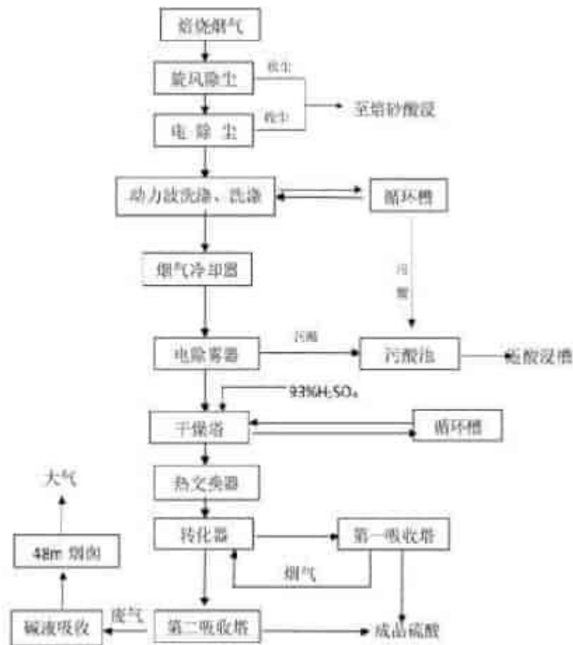
图 4.1-2 制酸系统生产工艺及污染物产出流程图
