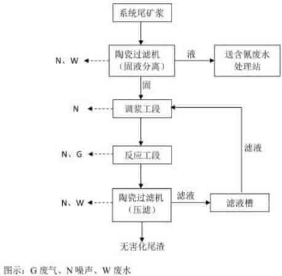
图 4.1-4 氰化尾渣工艺流程及产污环节示意图
