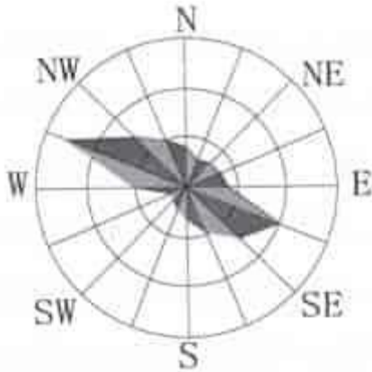
图 3.2-1 风向玫瑰图
