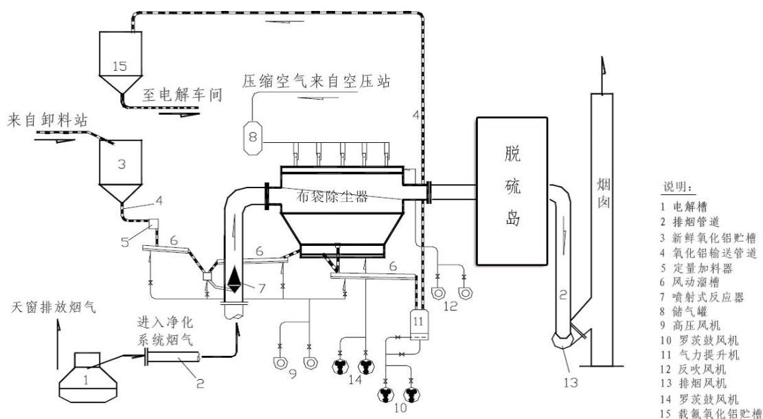
图 2-12 电解槽烟气净化工艺流程图
