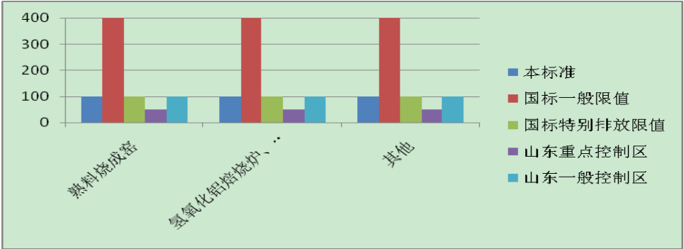
图 8-2 氧化铝厂二氧化硫标准限值对比
