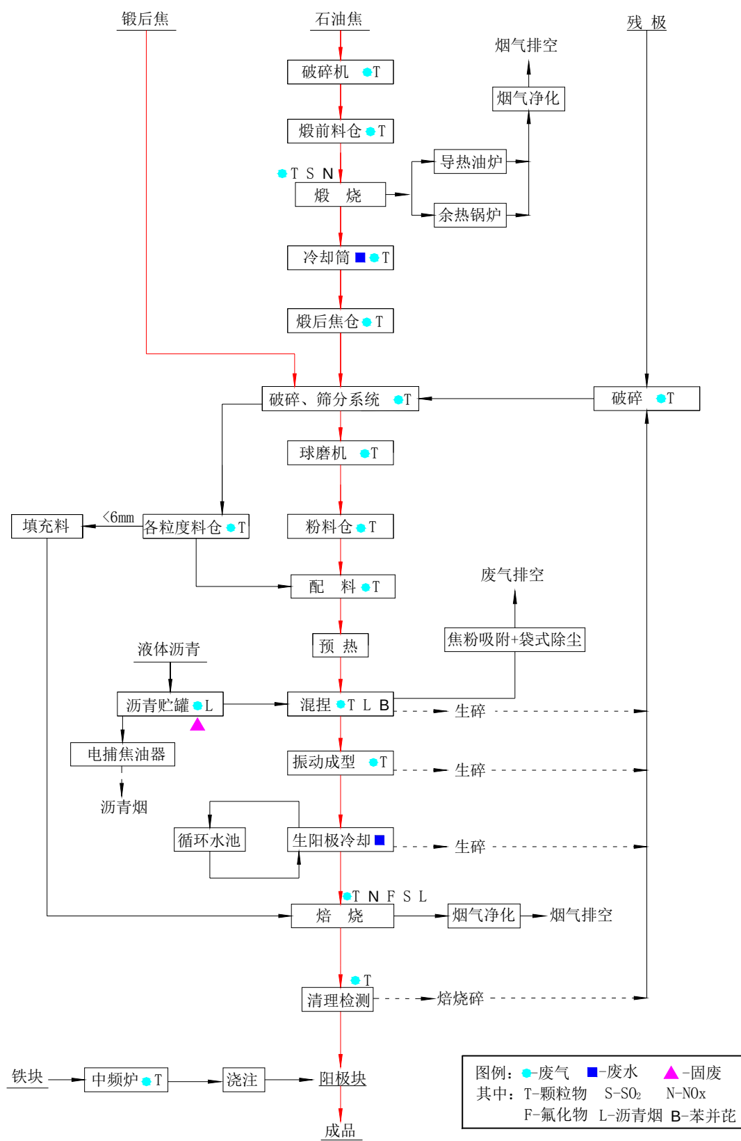
图 2-9 阳极炭素生产工艺流程及产污节点图
