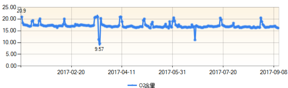
图 7-5 炭素焙烧工序烟气含氧量
