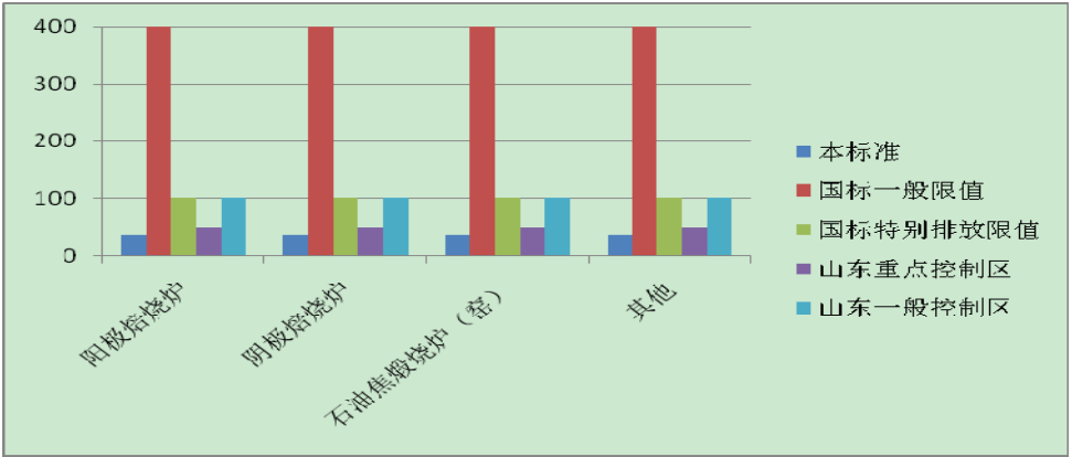
图 8-7 铝用炭素厂二氧化硫标准限值对比
