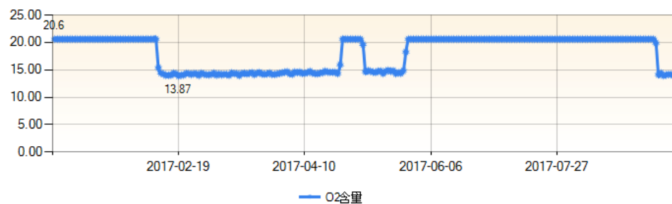
图 7-4 炭素煅烧工序烟气含氧量
