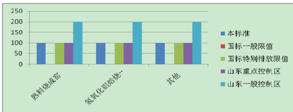
图 8-3 氧化铝厂氮氧化物标准限值对比
