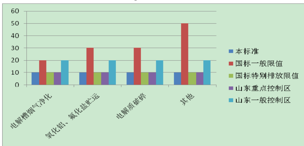
图 8-4 电解铝厂颗粒物标准限值对比
