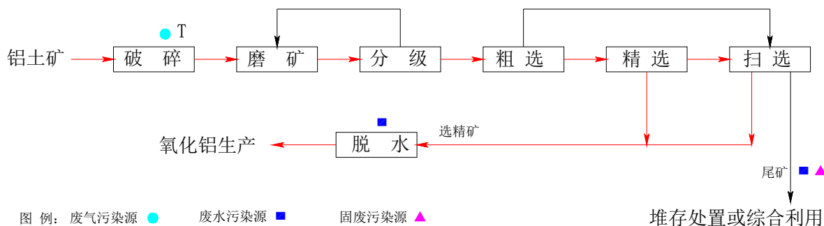
图 2-6 铝土矿选矿工艺流程及产污节点图
