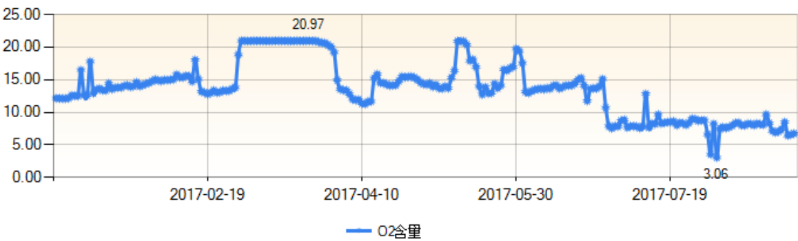
图 7-2 氧化铝焙烧炉烟气含氧量
