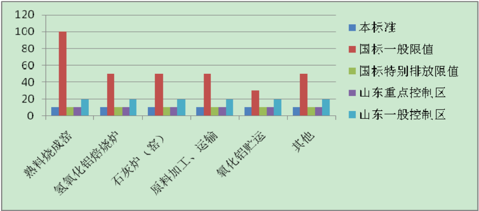
图 8-1 氧化铝厂颗粒物标准限值对比
