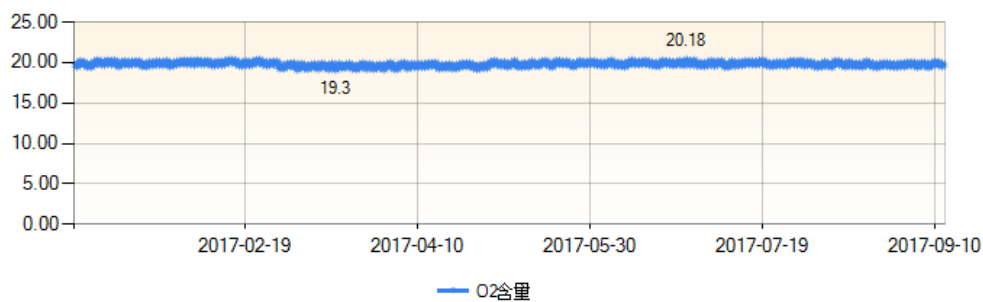
图 7-3 电解工序烟气含氧量
