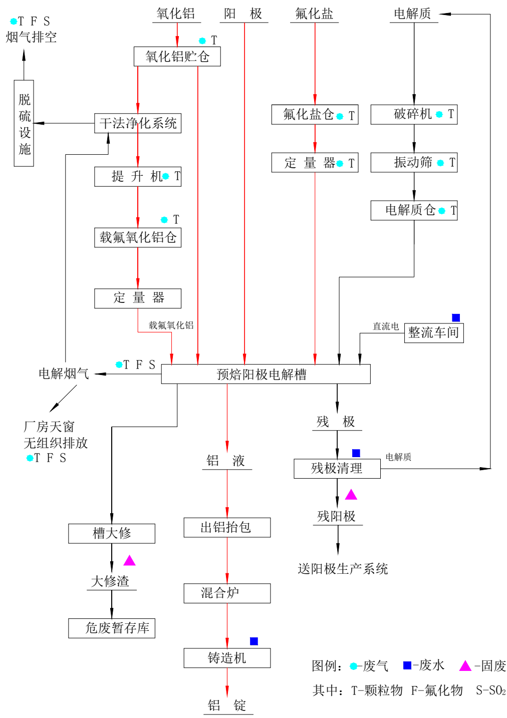
图 2-8 电解铝工艺流程及产污节点图
