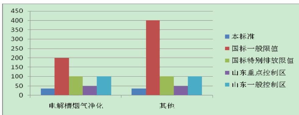
图 8-5 电解铝厂二氧化硫标准限值对比
