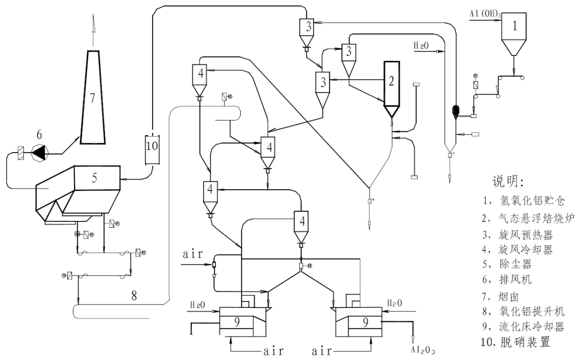
图 2-11 氢氧化铝焙烧炉烟气净化工艺流程图
